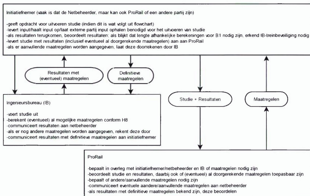
Figuur 2: Flowchart ten behoeve van EMC-detailstudie proces
